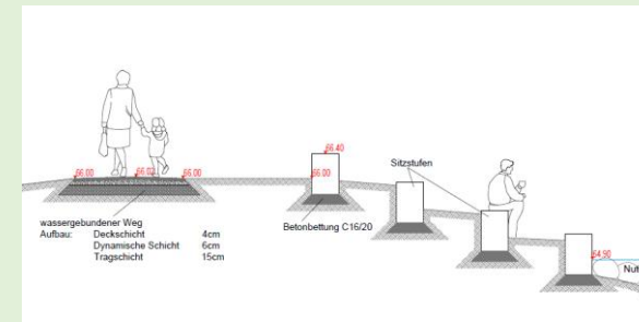
Schnitt Sitzstufen
