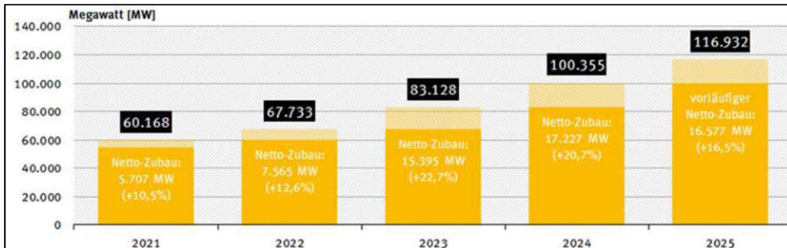
Abbildung 2: Netto-Zubau Photovoltaik der letzten 5 Jahre (Quelle: AGEE-STAT, STAND: 13.01.2026)
